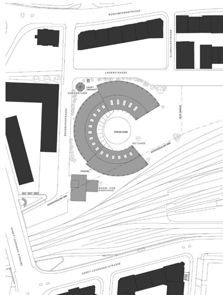
Lokremise mit Badhaus und Wasserturm (Situation)
